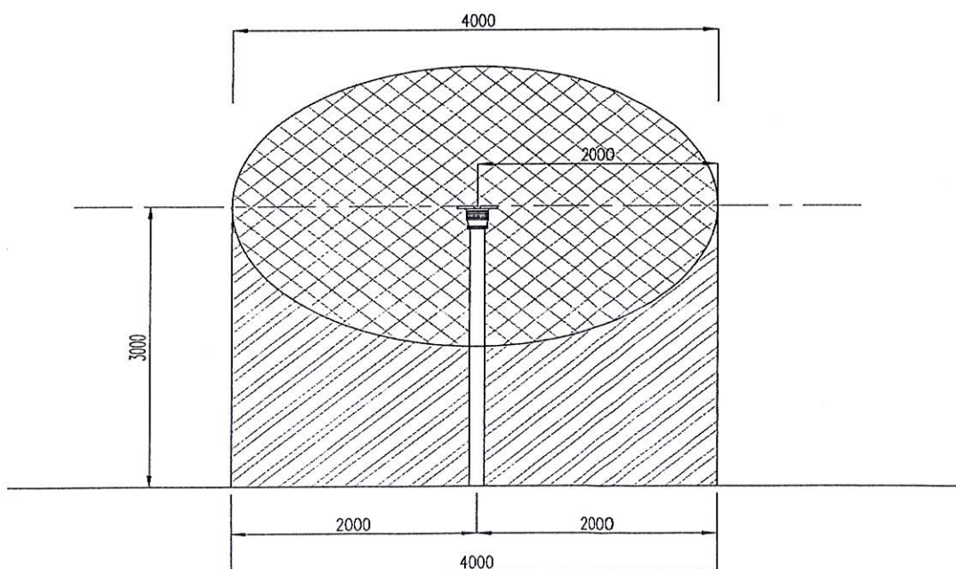
Hình 6: Vùng nguy hiểm cháy nổ của van thở khi không có thu hồi hơi.
